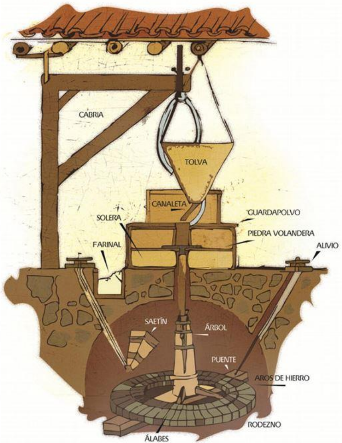
Partes de un Molino Hidráulico Harinero
